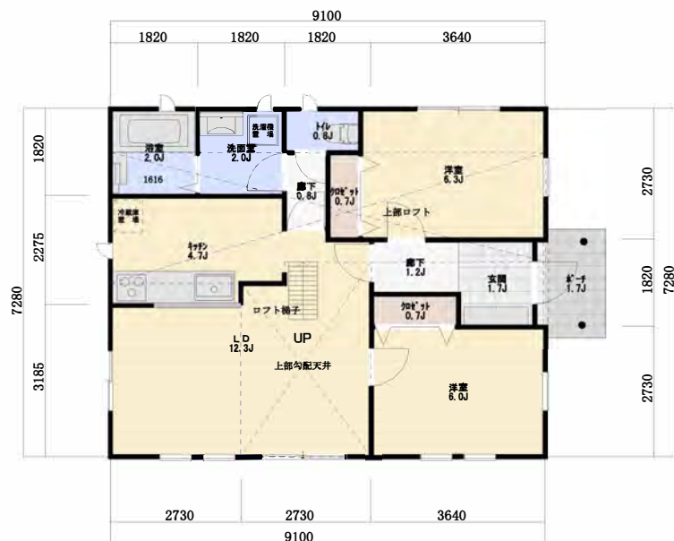
1 階平面図 9100
