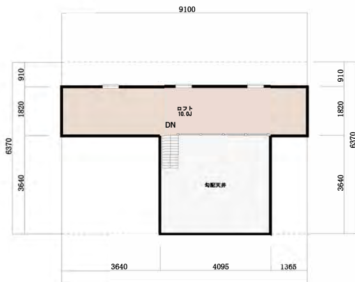
小屋裏平面図
