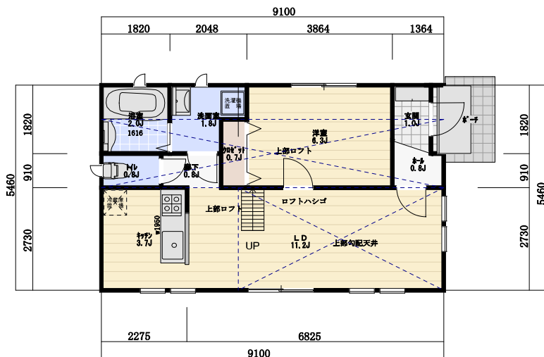
1階平面図
