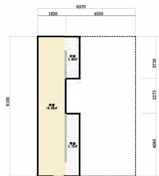
ロフト平面図
