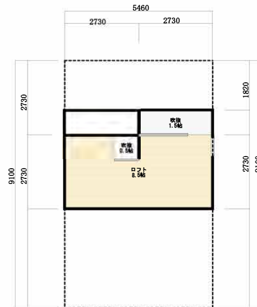
ロフト平面図
