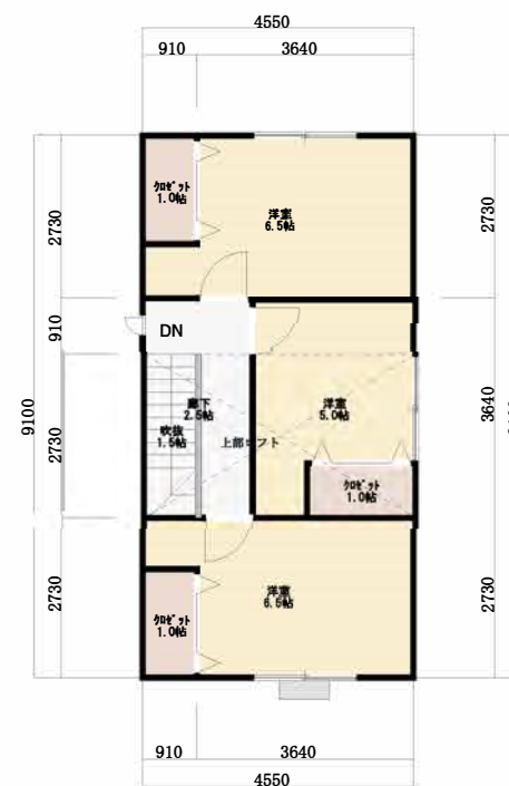
2階平面図
