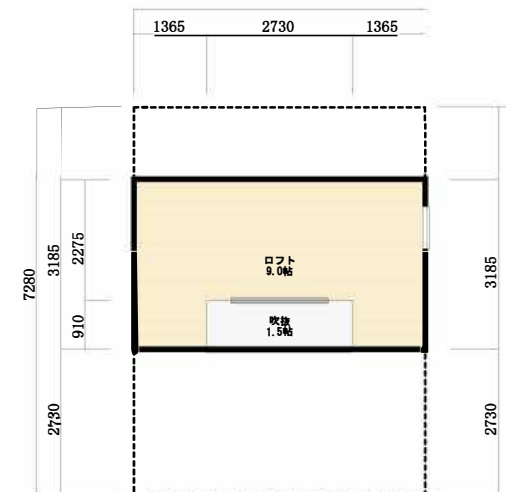
ロフト平 面図
