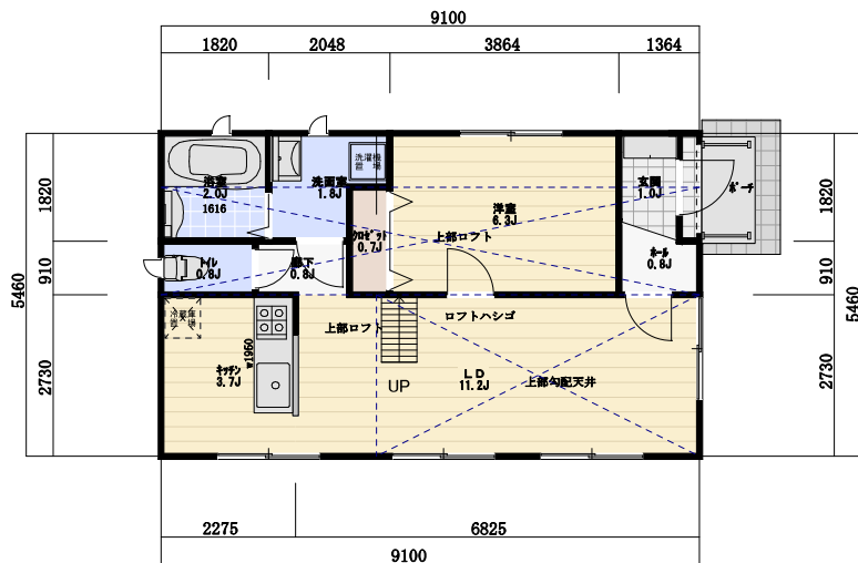
1階平面図
