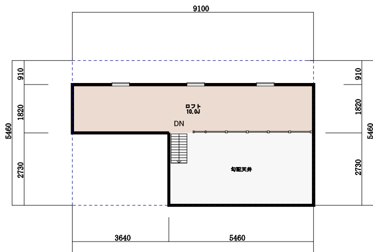
小屋裏平面図
